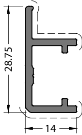
CODE / KOD 72ES-521-00 THEORETICAL WEIGHT kg/m TEORİK AĞIRLIK kg/m 0.277
