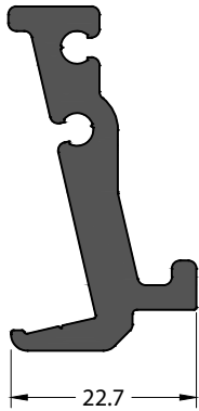
No visible surface. Görünen yüzeyi yoktur. CODE / KOD 09-903-00 THEORETICAL WEIGHT kg/m TEORİK AĞIRLIK kg/m 0.846
