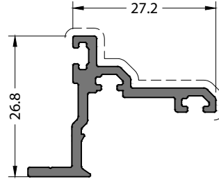
CODE / KOD 72ESHI-512-00 THEORETICAL WEIGHT kg/m TEORİK AĞIRLIK kg/m 0.365
