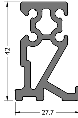
No visible surface. Görünen yüzeyi yoktur. CODE / KOD 72ES-901-00 THEORETICAL WEIGHT kg/m TEORİK AĞIRLIK kg/m 0.641
