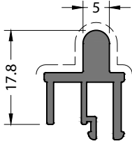
CODE / KOD 72ES-511-00 THEORETICAL WEIGHT kg/m TEORİK AĞIRLIK kg/m 0.284
