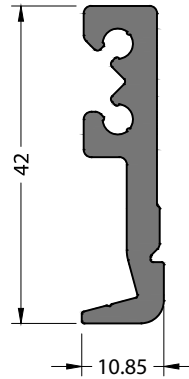
No visible surface. Görünen yüzeyi yoktur. CODE / KOD 72ES-901-00 THEORETICAL WEIGHT kg/m TEORİK AĞIRLIK kg/m 0.641
